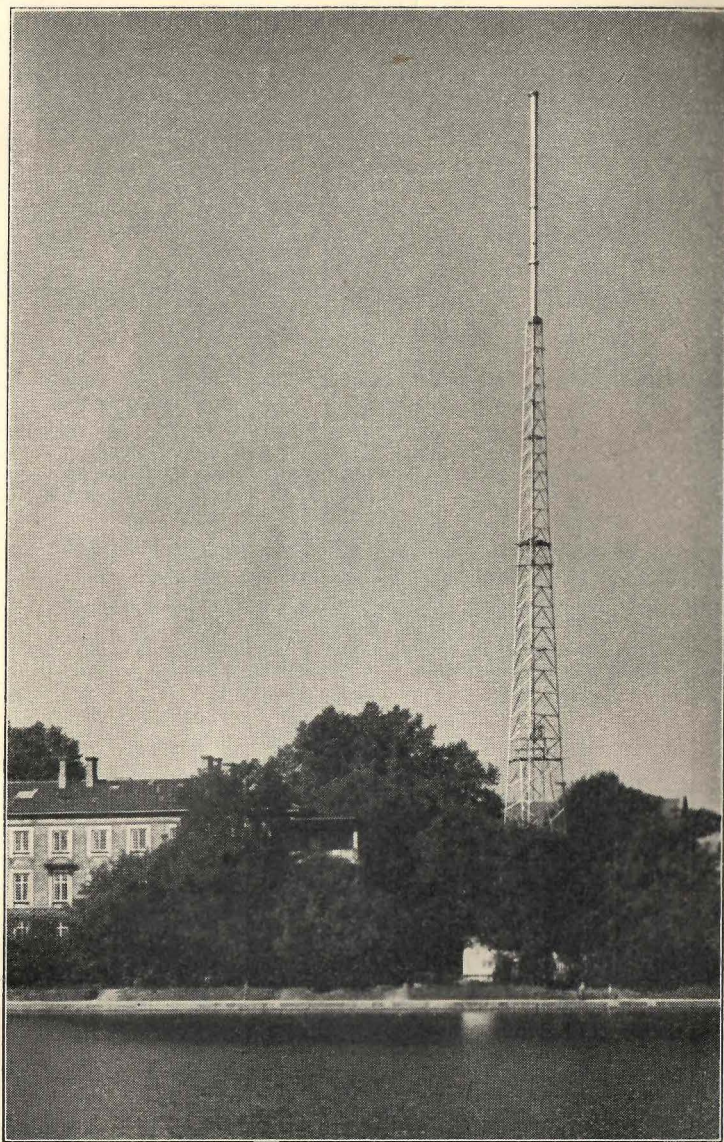
Antenneanlægget ved den nye radiofonistation ved Nørre hospital i København.
