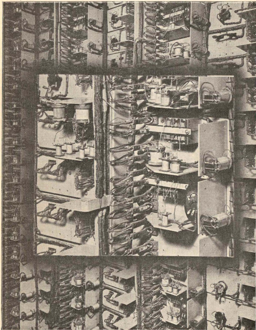
Udsnit af Forsterkeranlægget paa Statstelefonkontoret i København (Kunstledningsstel).
