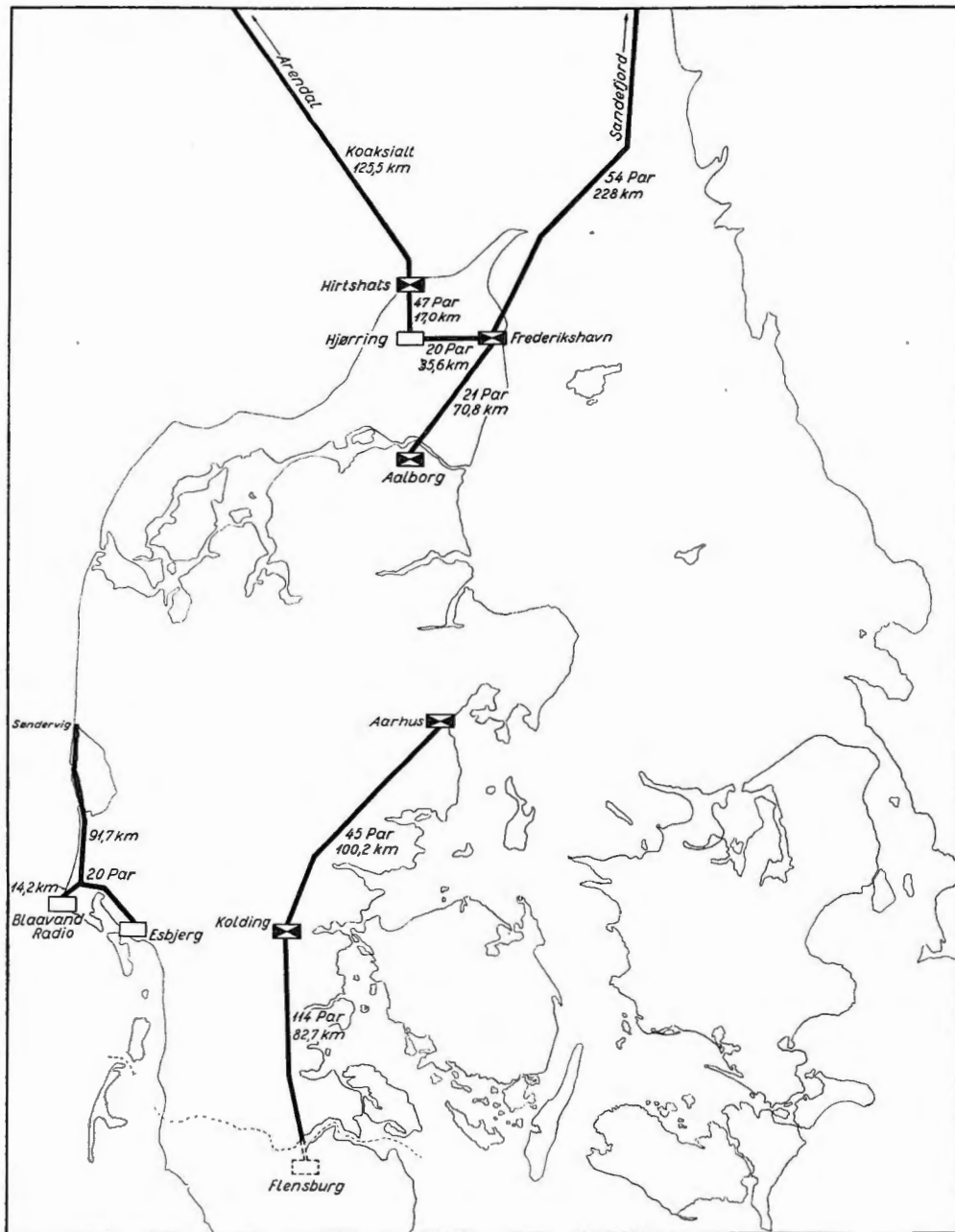
Kort over de fra den tyske Værnemagt overtagne Kabler og Forstærkerstationer.
