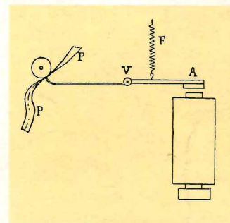
Morseapparatets princip: P er papirstrimmelen, V er vægtstangen, F er fjederen og A er ankeret.
